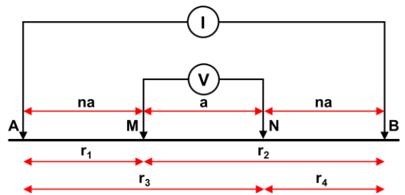
Gambar 2. Susunan elektroda konfigurasi Schlumberger
